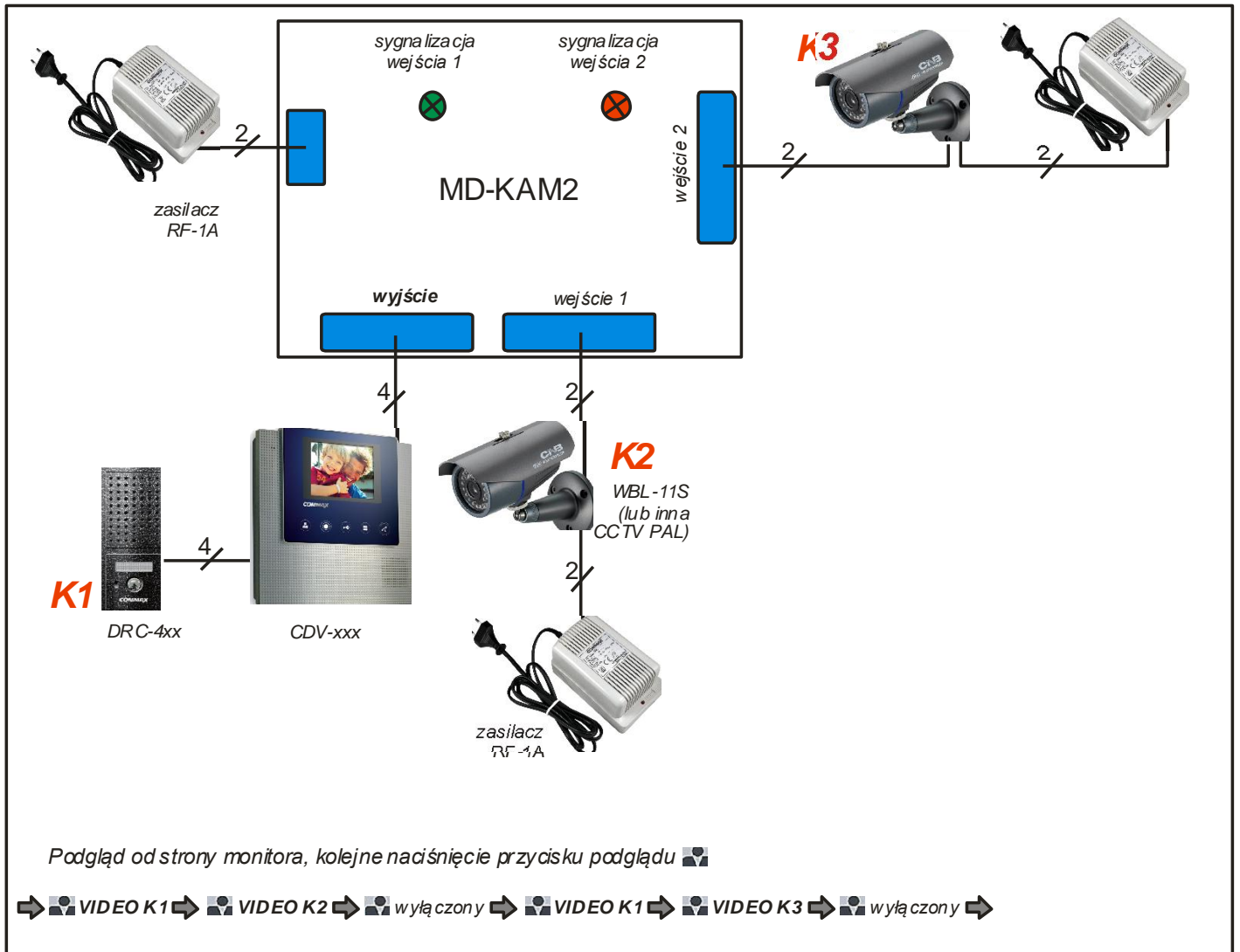
Rys 4 Przykład podłączenia
