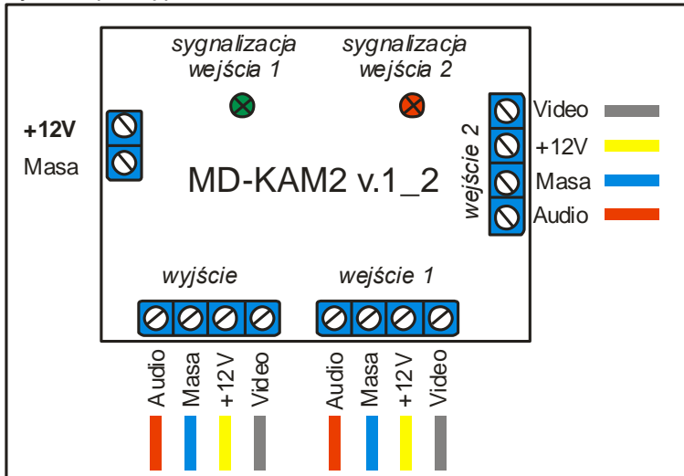
Rys 1. Opis wyprowadzeń
