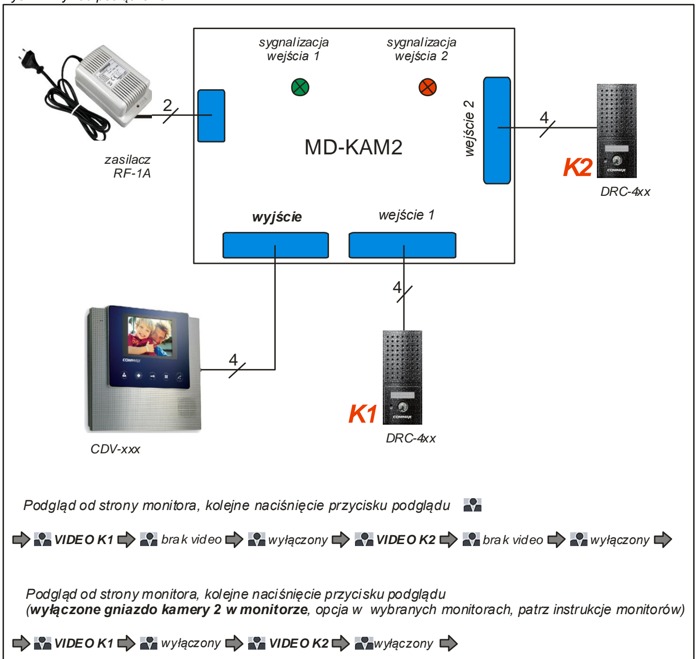
Rys 2. Przykład podłączenia
